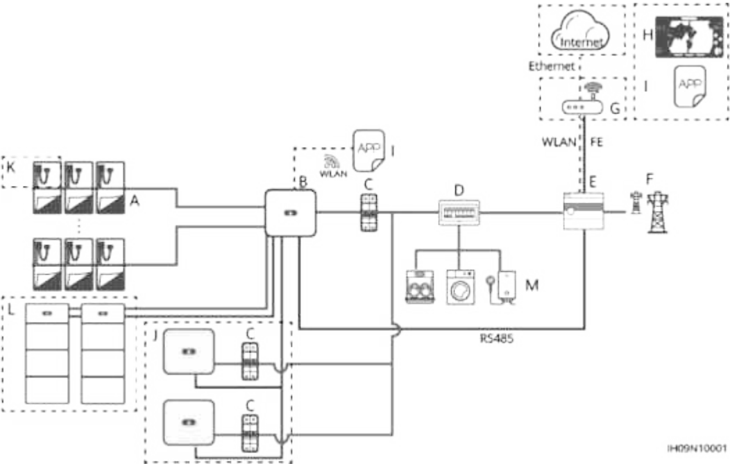
Figure 2-2 Mise en réseau du SmartAssistant (les composants dans les encadrés en pointillés sont facultatifs)
