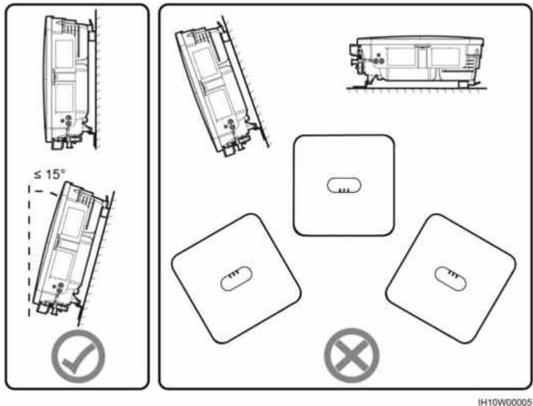
Figure 4-5 Angle d'installation
