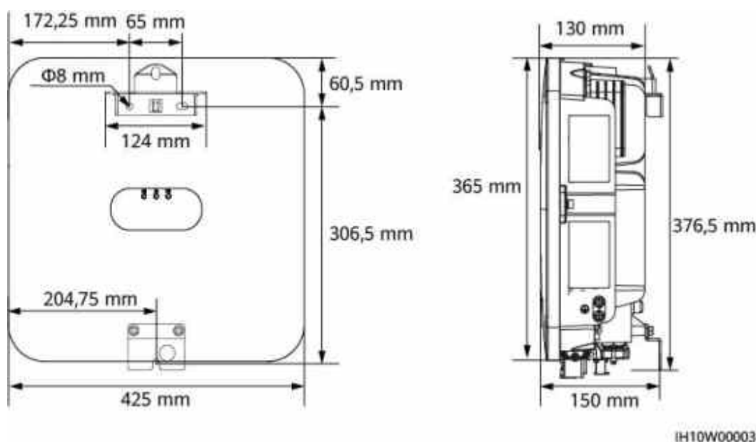
Figure 4-1 Dimensions du support de montage
