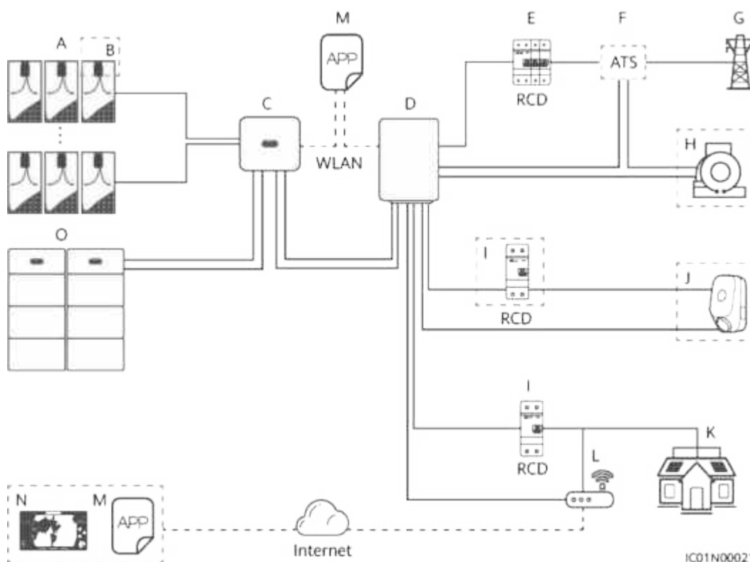
Figure 2-4 Mise en réseau du SmartGuard (les composants dans les encadrés en pointillé sont facultatifs)
