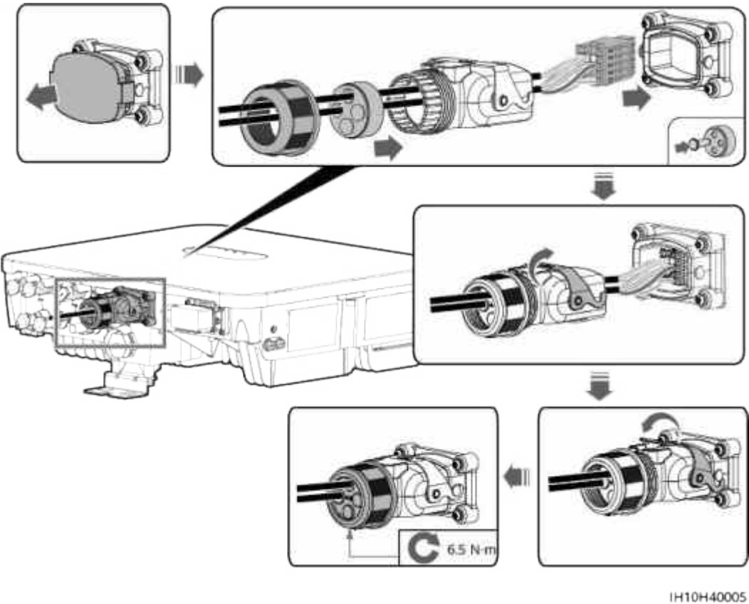
Figure 5-31 Fixation du connecteur du câble de signal
